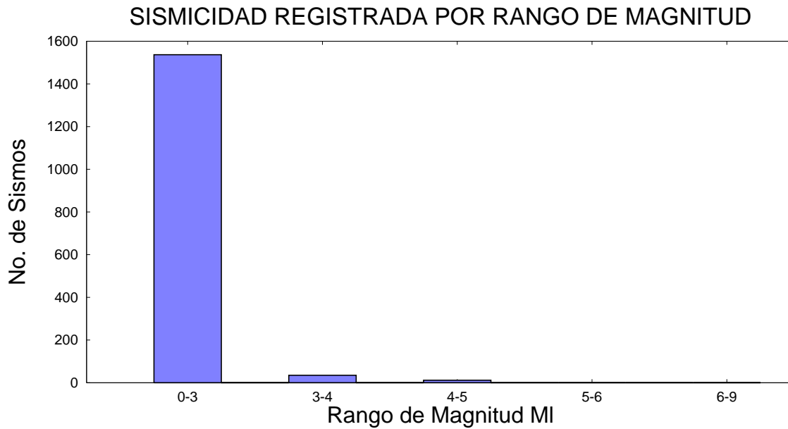
Figura 4: Número de sismos registrados por rango de magnitud, diciembre de 2016
